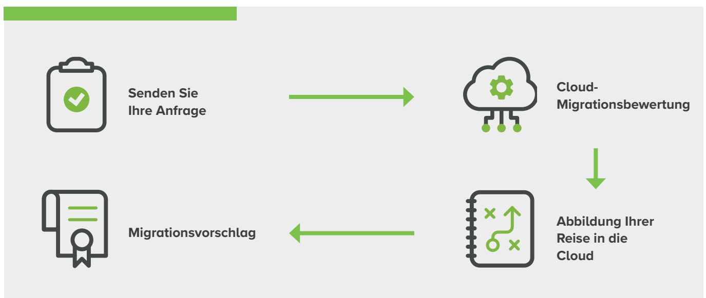
Abbildung 1: Der Cloud-Migrationsbewertungsprozess
